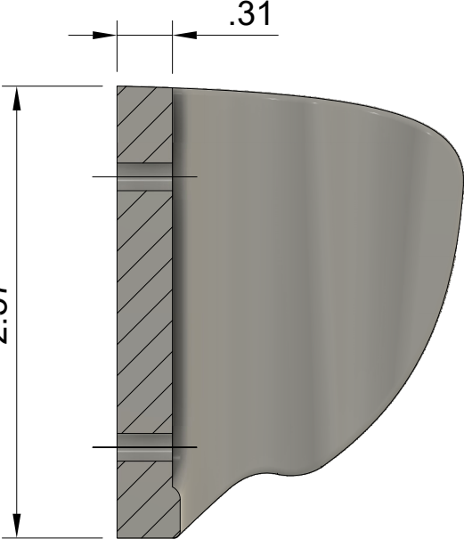
A-A (1:1)
